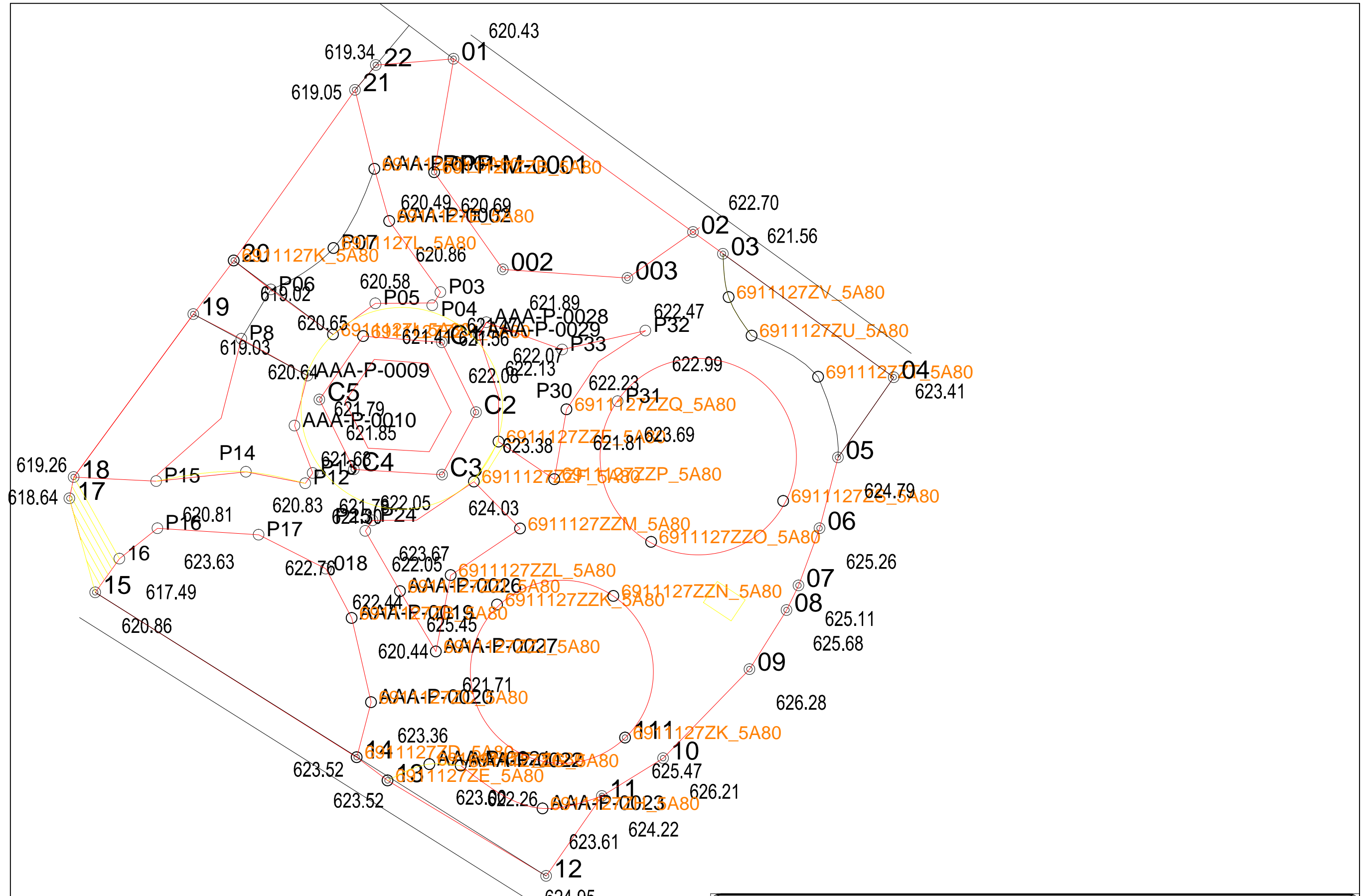
PLANIALTIMETRICO BRAÇA BRASIL - SIQUEIRA CAMPOS S/ ESCALA
