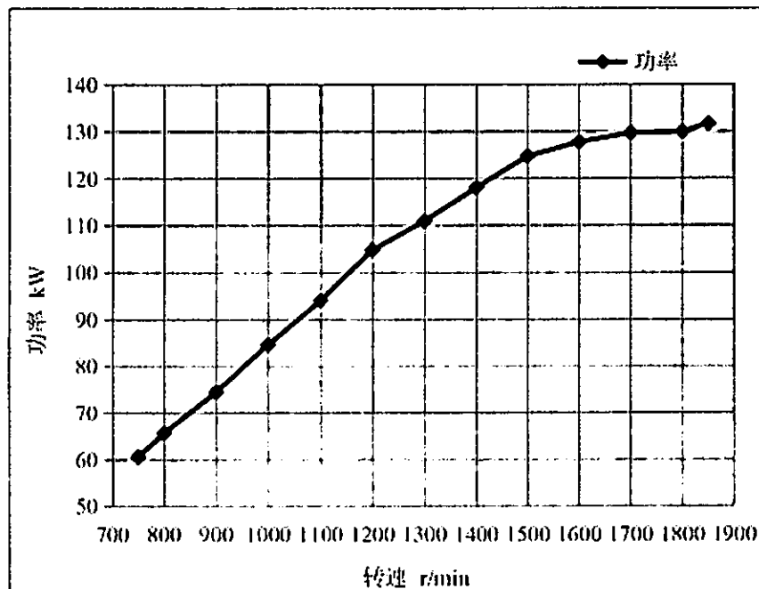
Curva de variação de potência com rotação do motor
