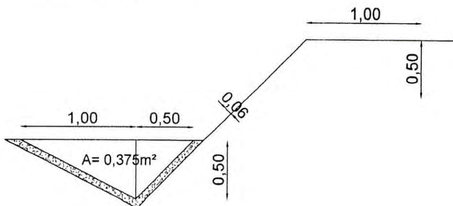
SARJETA EM CORTE 150x50 CONCRETO f_{ck} = 20\text{MPa}
