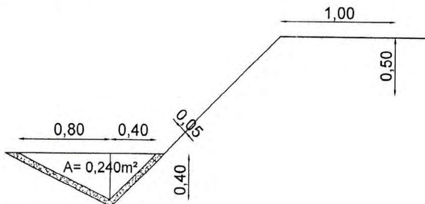
SARJETA EM CORTE 120x40 CONCRETO f_{ck} = 20\text{MPa}
