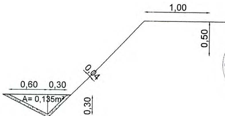
SARJETA EM CORTE 120x40 CONCRETO f_{ck} = 20\text{MPa}
