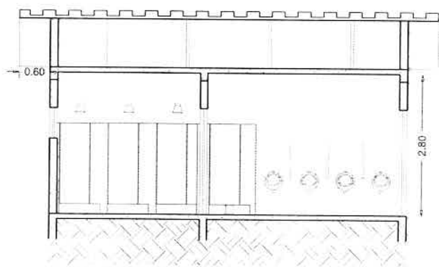
03 Corte BB Bwc Fem. ESC.: 1/50
