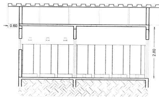
02 Corte AA Bwc Fem. ESC.: 1/50
